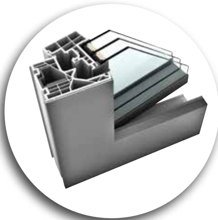
Widok okna z zewnątrz - skrzydło szklane
